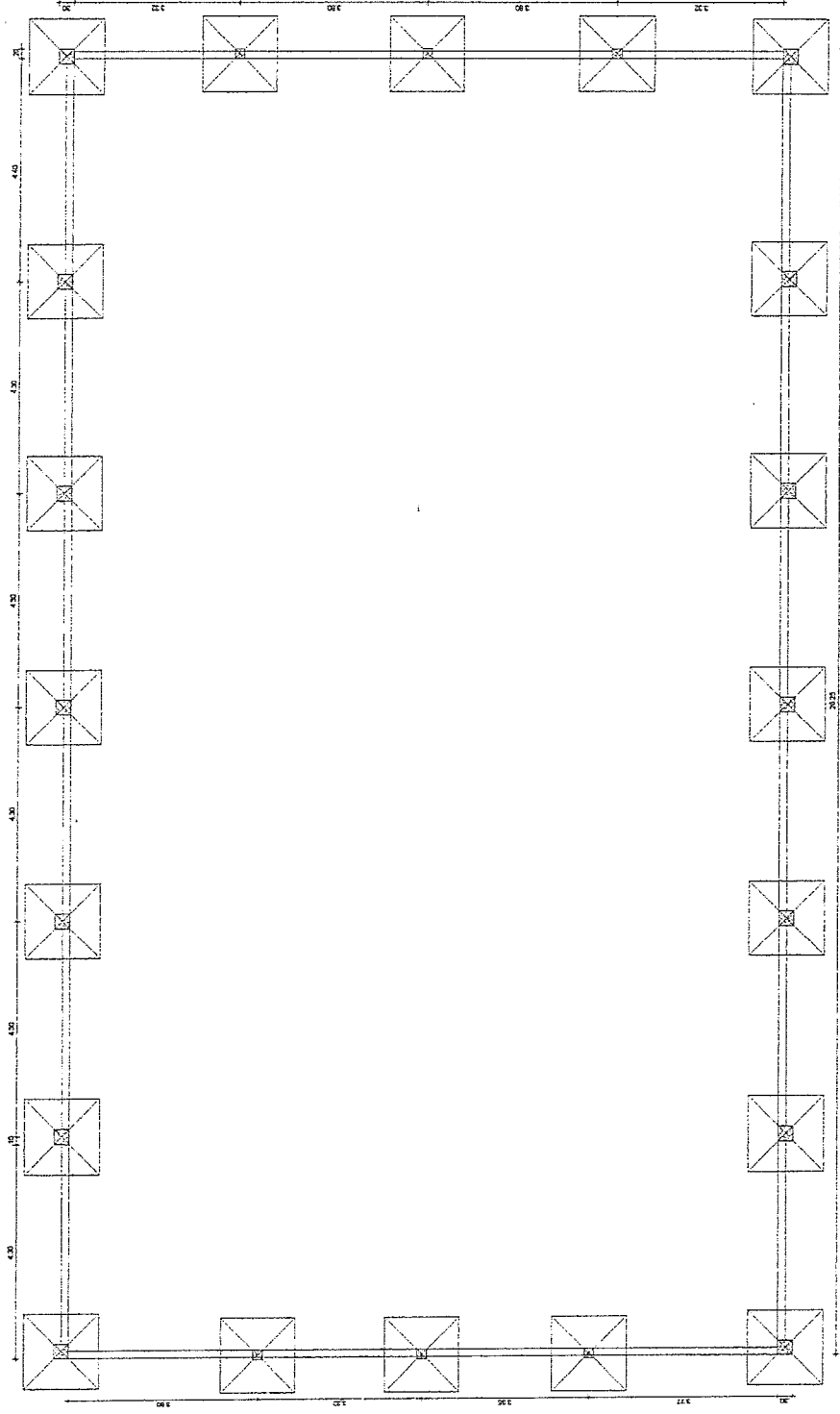
1 PLANTA BASES ESCALA 1:50
