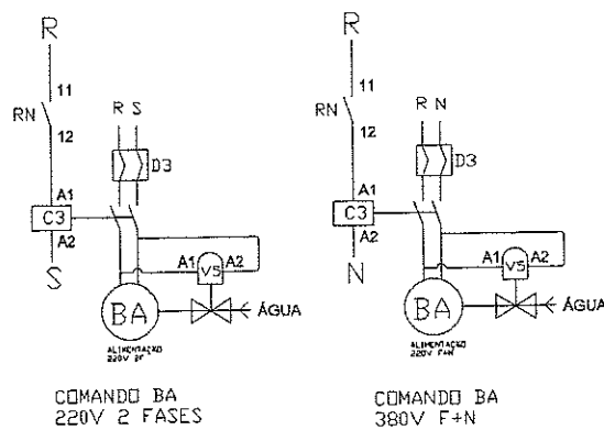
Fig. 08. Diagrama elétrico de fechamento da porta.
