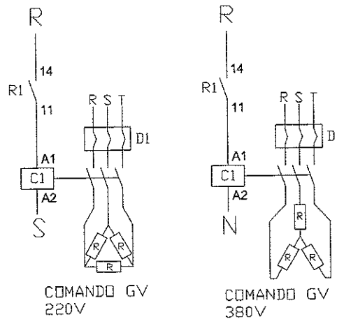
Fig. 07. Diagrama elétrico do gerador de vapor.
