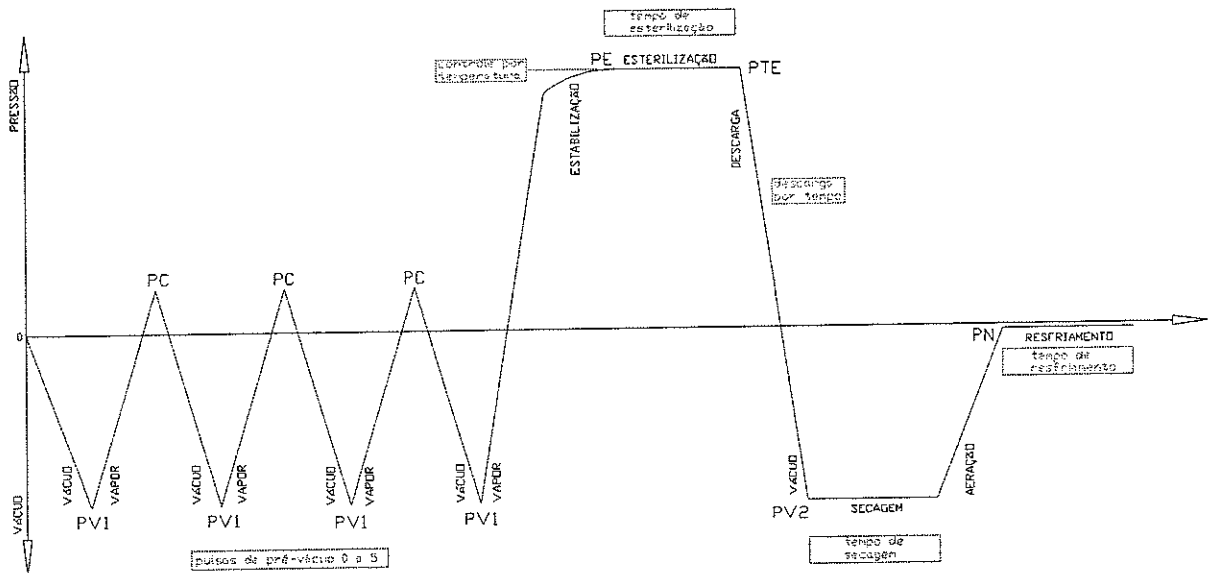
Fig. 56. Diagrama de ciclo – pressão.
