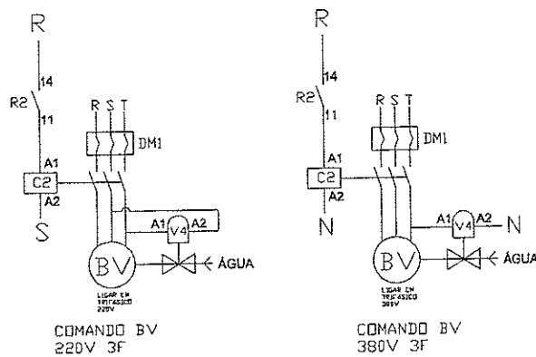
Fig. 09. Diagrama elétrico de acionamento da bomba de vácuo.
