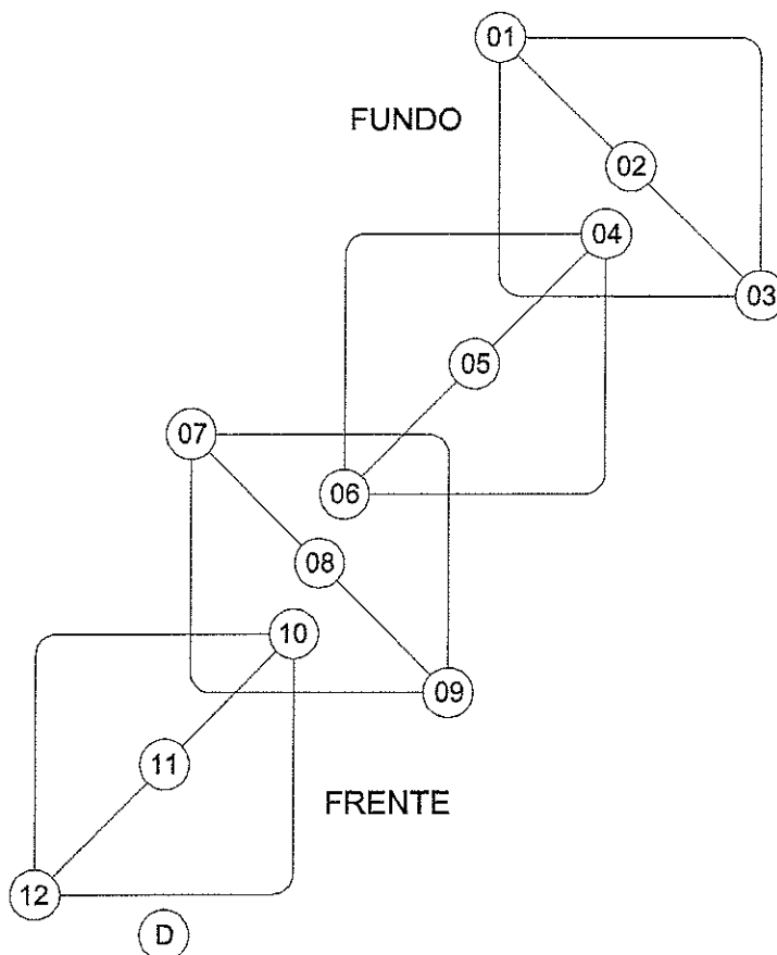
Fig. 07. Posicionamento recomendado para os sensores de temperatura.
