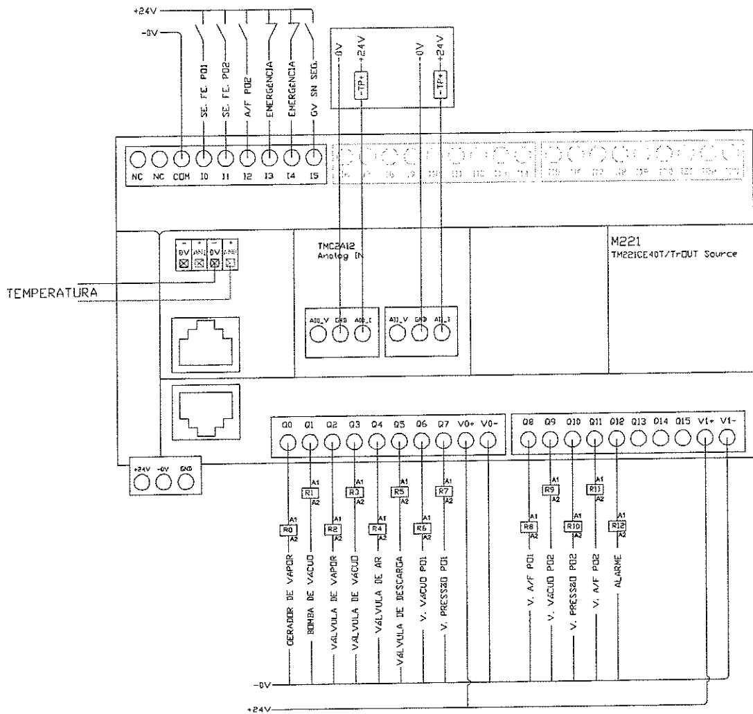
Fig. 06. Diagrama elétrico do controlador.
