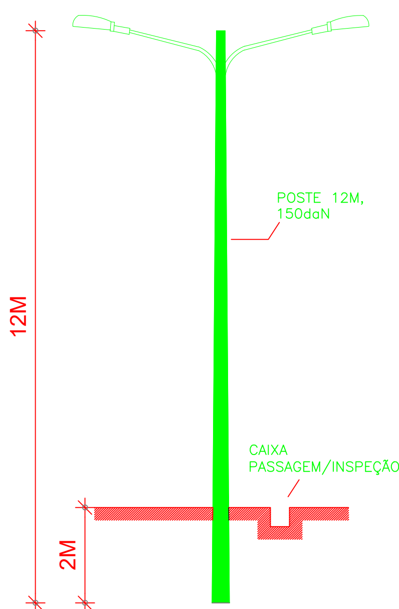
08 DETALHE POSTE SEM ESCALA
