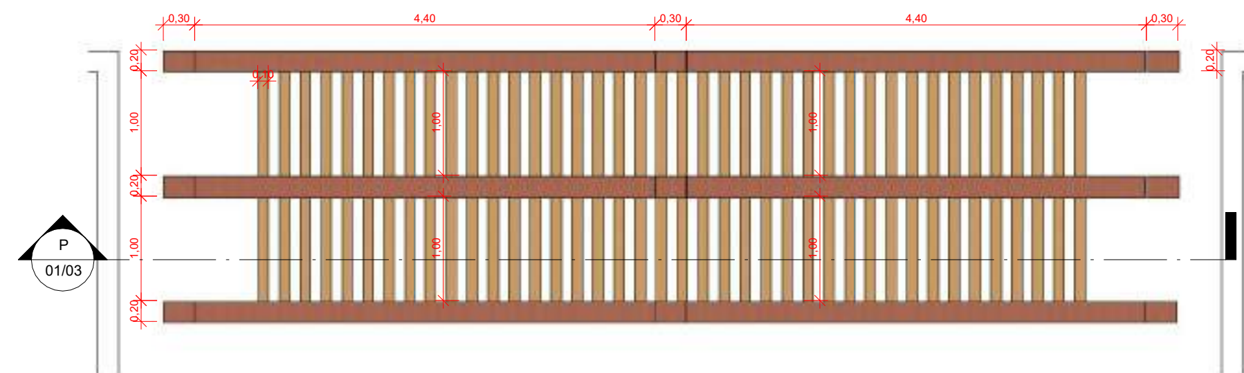
DETALHAMENTO PÓRTICO
