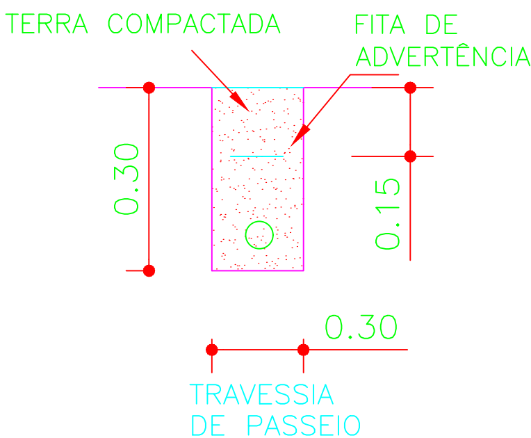
06 DETALHE DE TRAVERSIA SEM ESCALA
