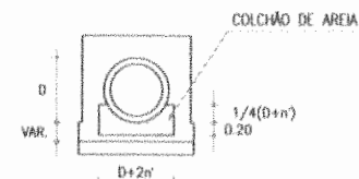
CORTE BB
